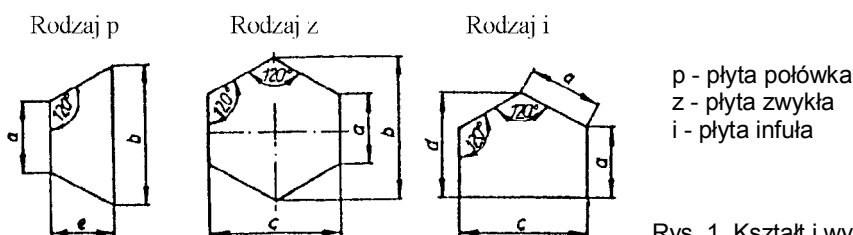
Rys. 1. Kształt i wymiary płyt betonowych
